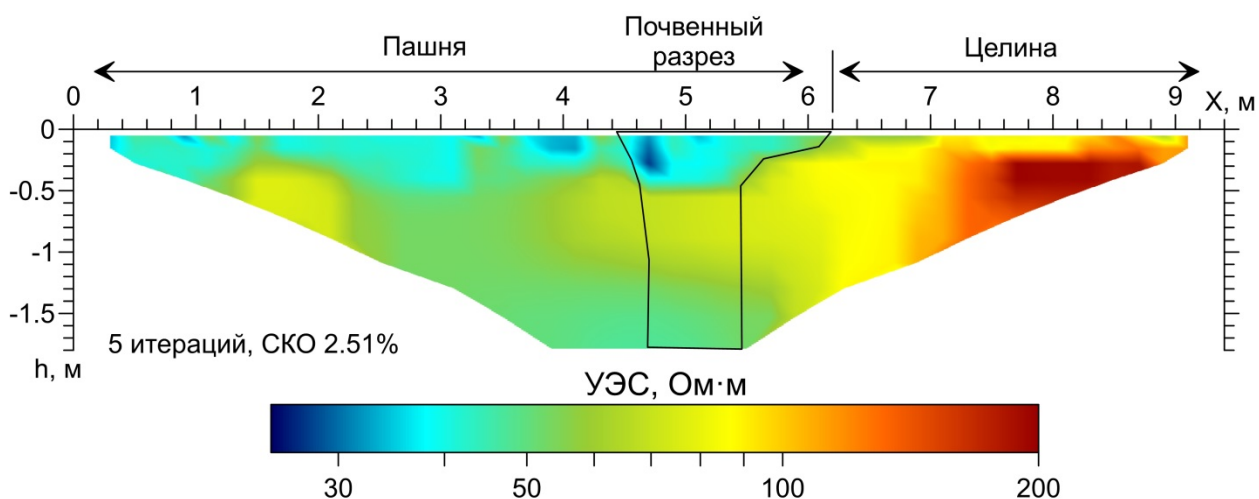
Рисунок 8. Геоэлектрический разрез на ключевой площадке АК (аккумулятивная позиция катены) по данным электротомографии.
