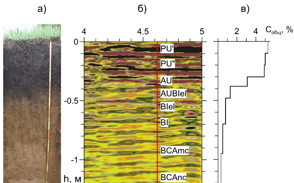
Рисунок 4. Сопоставление строения почвенного профиля (а), георадиолокационного разреза (б) и распределения общего углерода по глубине (в) на ключевой площадке EL (элювиальная позиция катены).
