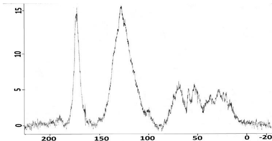
Рисунок 9. ^{13}\text{C} ЯМР спектры ГК чернозема КА обыкновенного в нативных условиях без выхода водорода (фон).
