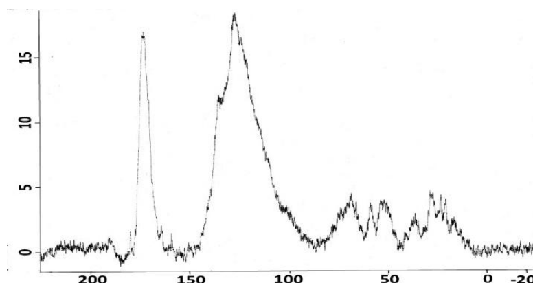
Рисунок 8. ^{13}\text{C} ЯМР спектры ГК чернозема обыкновенного в нативных условиях западины с потоком водорода.
