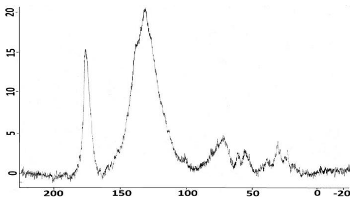
Рисунок 10. ^{13}\text{C} ЯМР спектры ГК чернозема обыкновенного в модельном опыте 3 с пропускаянием водорода.
