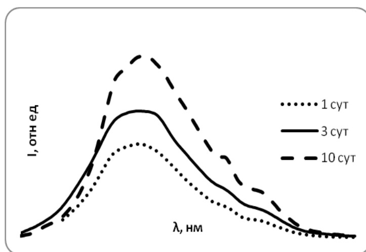
Рисунок 2. Спектры флуоресценции образца 3-1 с разной продолжительностью высушивания, I – интенсивность излучения, \lambda_{\text{возб}} = 260 нм.
